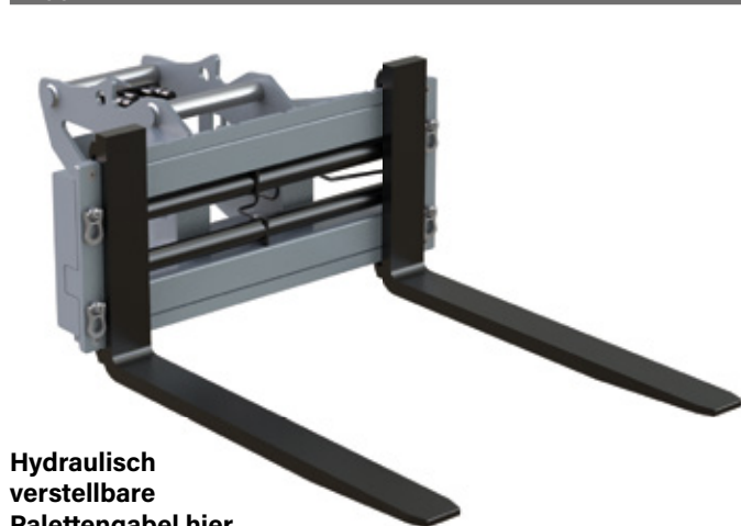
Hydraulisch verstellbare Palettengabel hier am zylinderlosen NOX Tiltrotator
